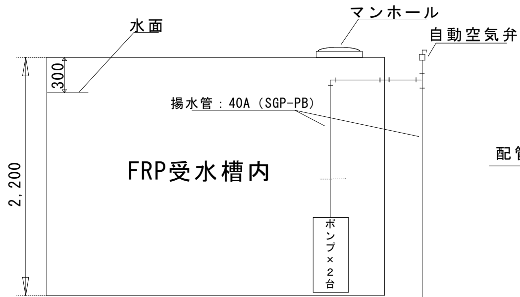
FRP受水槽側面図（標準） S=1/X
