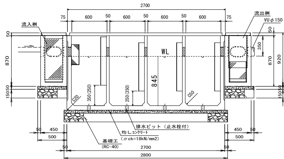
正面断面図
