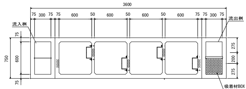
槽内平面図
