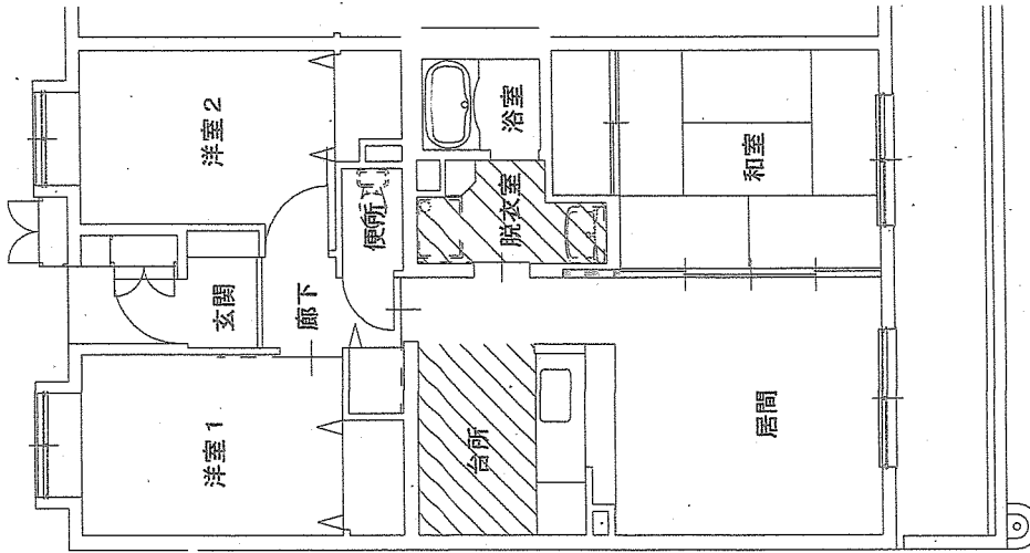
阿南宿舍 1号棟 3LK室 平面図
