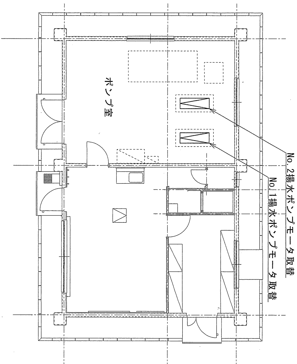
193号建物平面図 S=1/100
