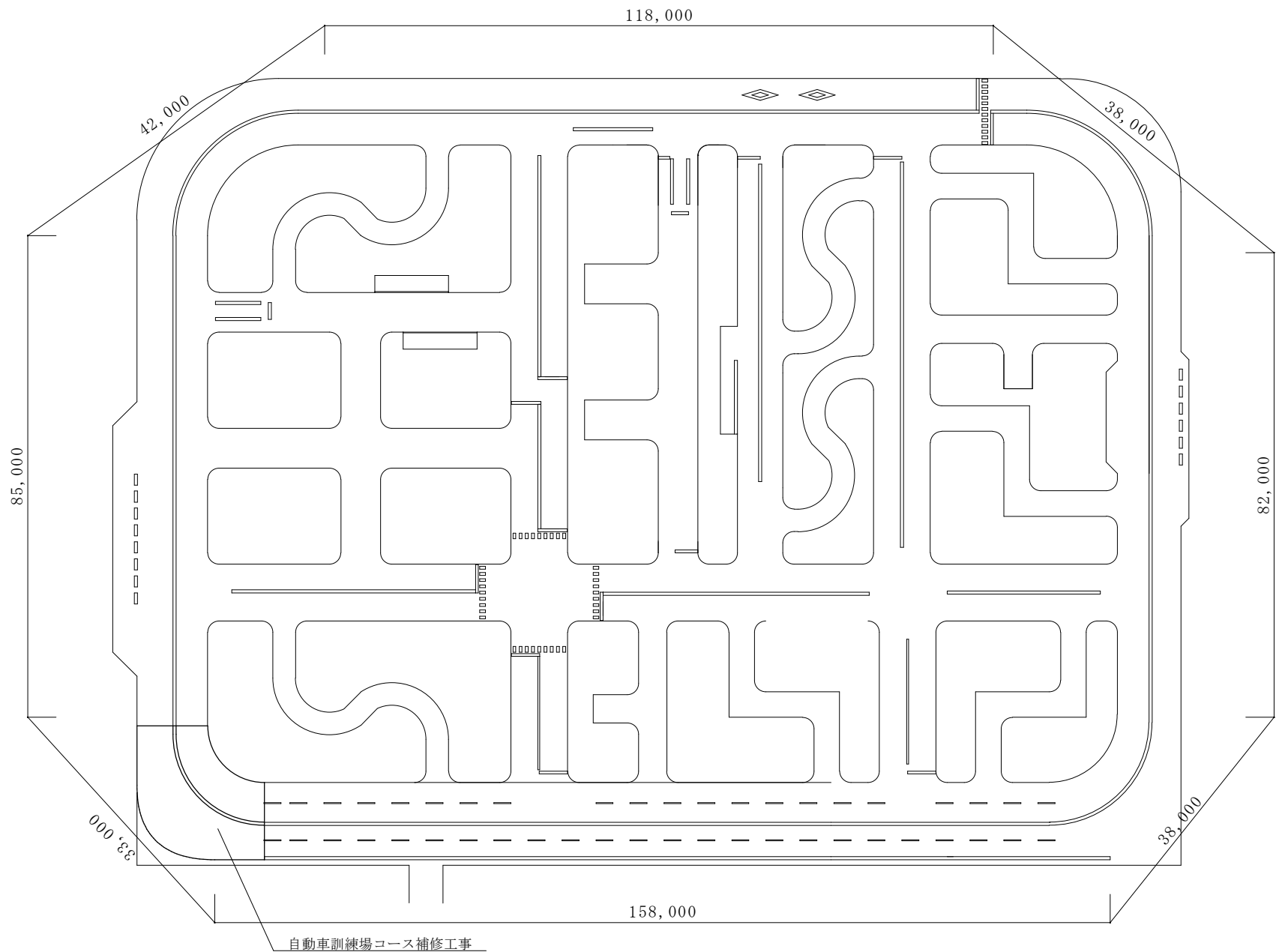
自動車訓練場平面図 S = 1 : 1 0 0 0
