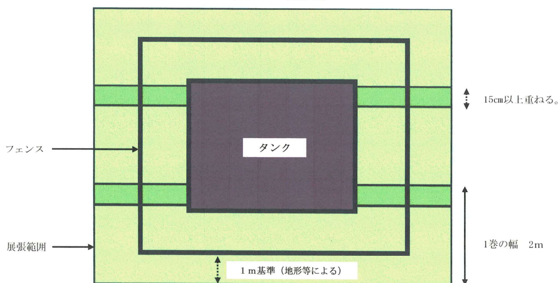
防草シート展張要領
