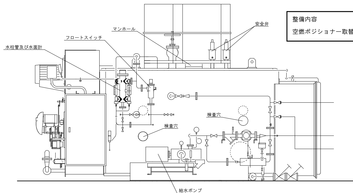
No. 1、2ボイラー側面図 S=1/30
