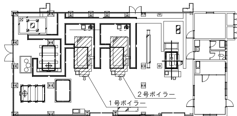
ボイラー室平面図 S=1/200
