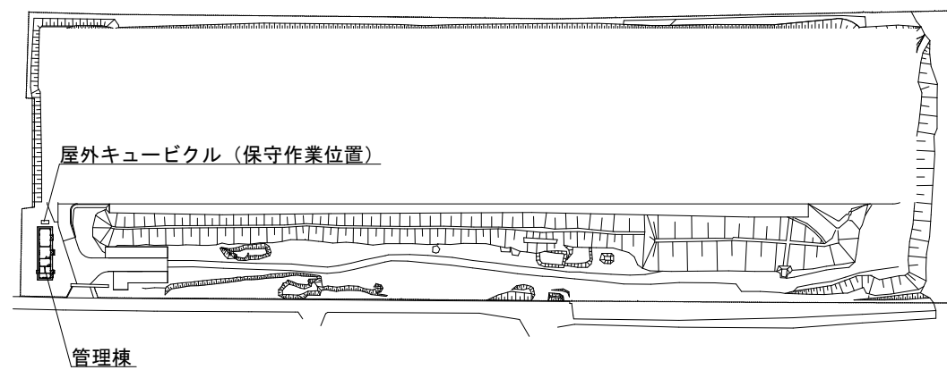
米子射撃場配置図
