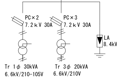
米子射場単線結線図
