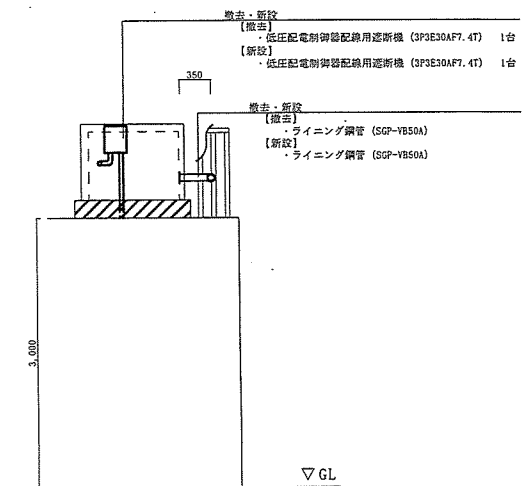
B面立面図
