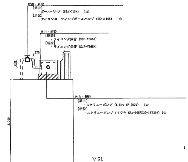
A面立面図
