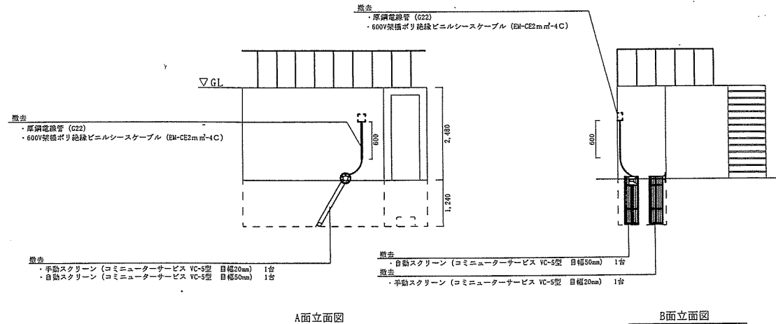
スクリーン施工箇所撤去立面図 S=1/100
