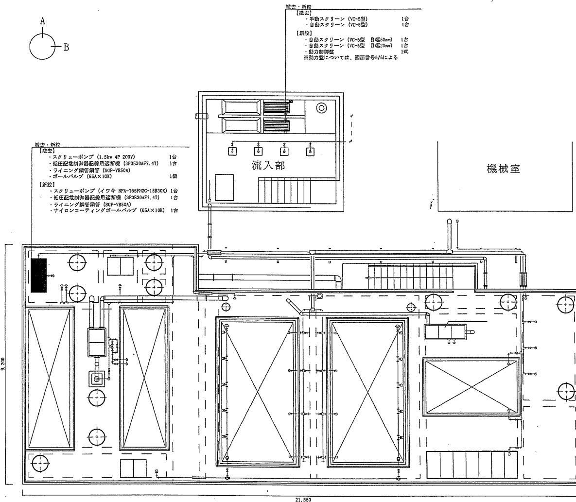
浄化槽平面図 S=1/100
