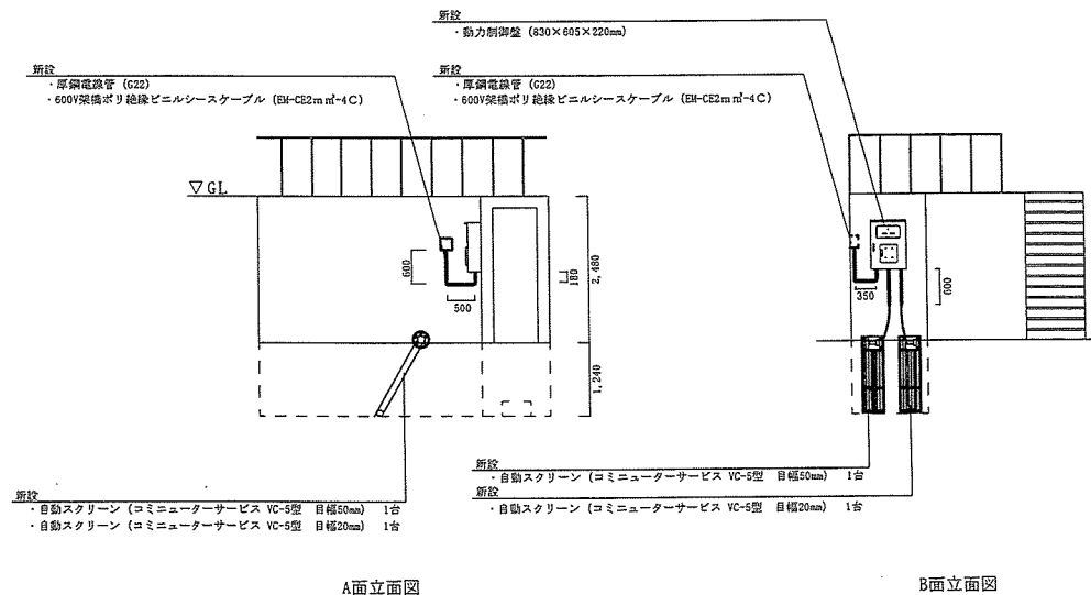
スクリーン施工箇所新設立面図 S=1/100
