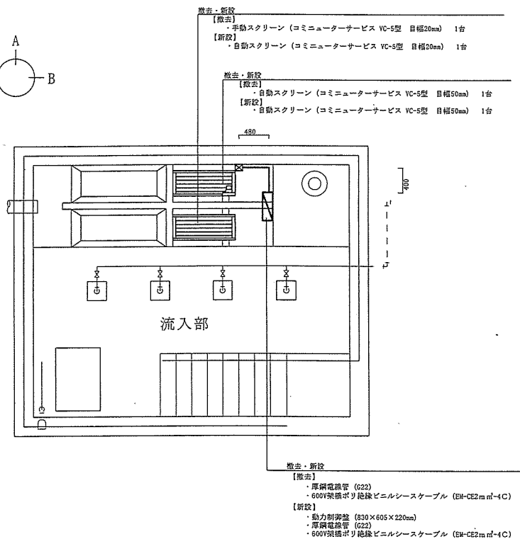
スクリーン施工箇所平面図 S=1/60
