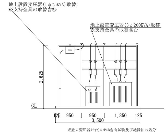
工事場所⑦ 立面図 S=1/80
