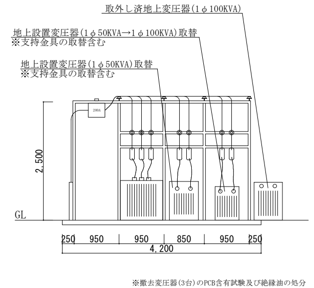
工事場所④ 立面図 S=1/80
