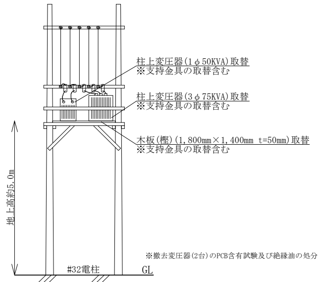
工事場所⑤ 立面図 S=1/120
