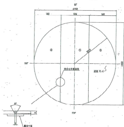
底板割付図 S=1:30
