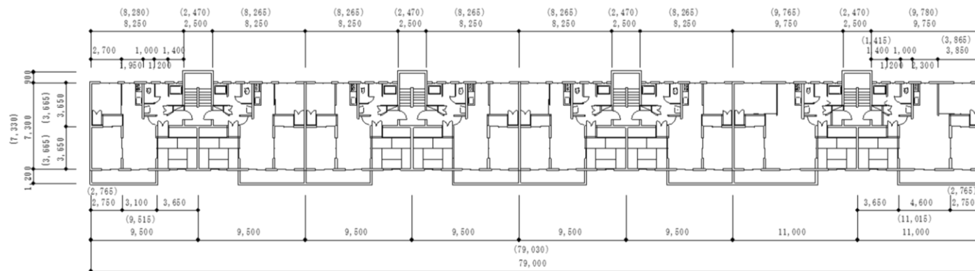
春日井宿舎 3 号棟平面図（各階） S=1/400
