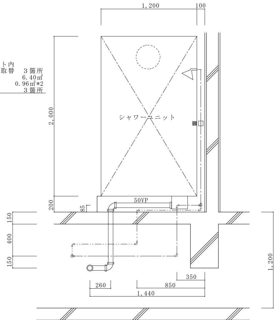
6 1 号隊舎シャワー室立面図 S=1/20
