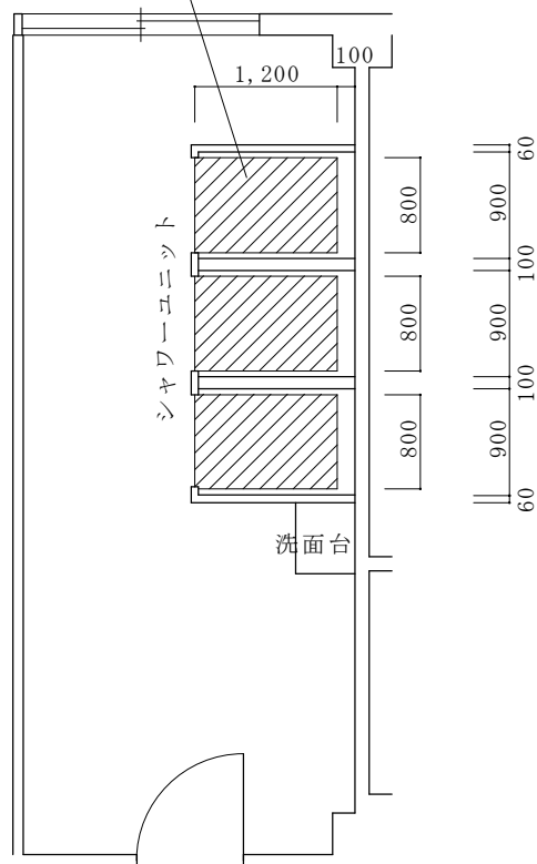
61号隊舎シャワー室平面図 S=1/50
