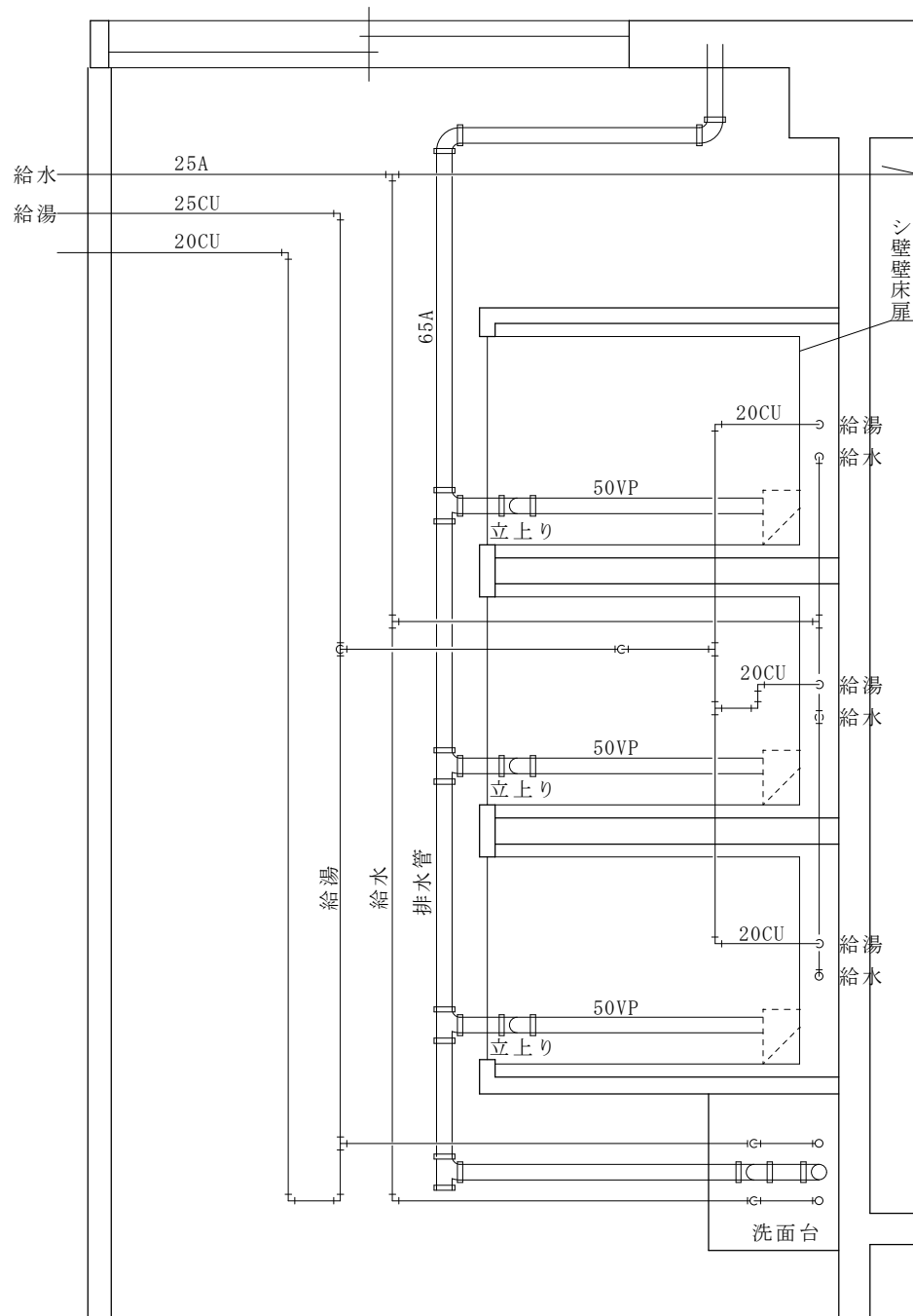
6 1 号隊舎シャワー室配管図 S=1/20
