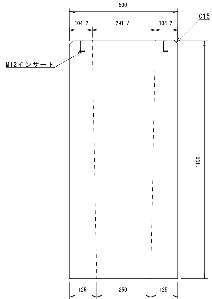
側 面 図
