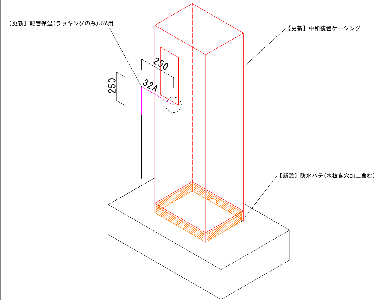
中和装置ケーシング 透視図
