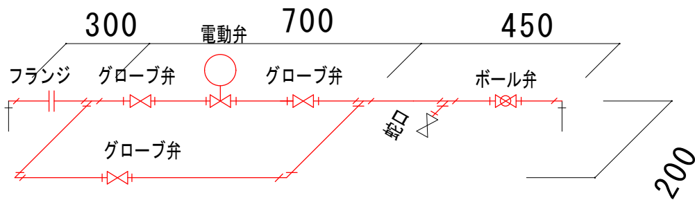
電動弁装置 透視図
