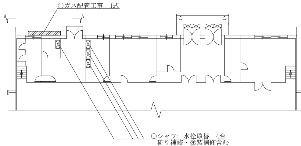
121号建物平面詳細図 S=1:Free
