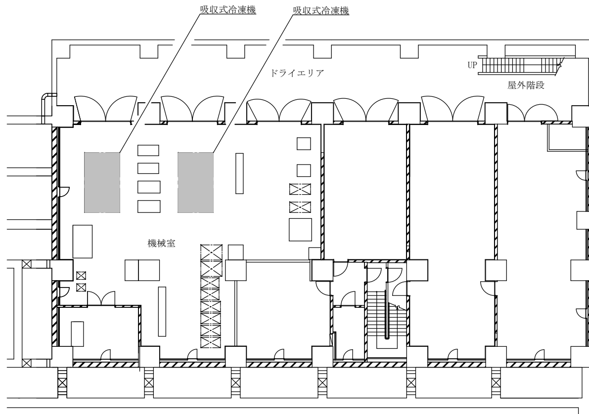
1号建物地階平面図 S = 1 / 2 5 0
