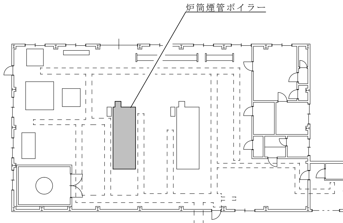
57号建物地階平面図 S = 1 / 2 5 0
