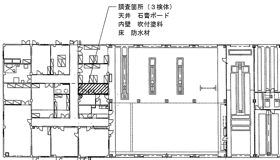
149号整備工場1階平面図
