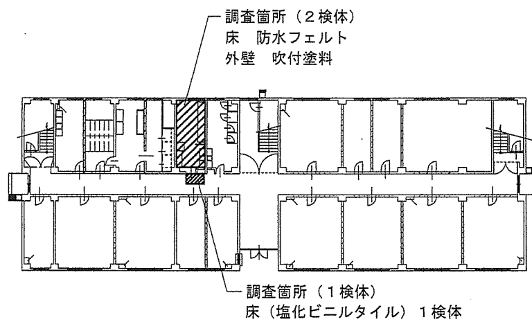
130号隊舎1階平面図
