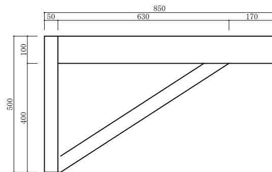
架台側面図 S=1/10
