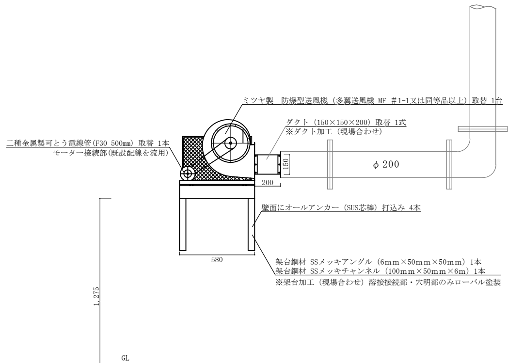
送風機正面図（東面） S=1/20
