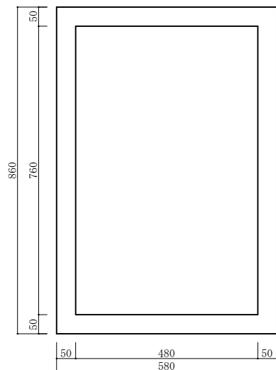
架台平面図 S=1/10
