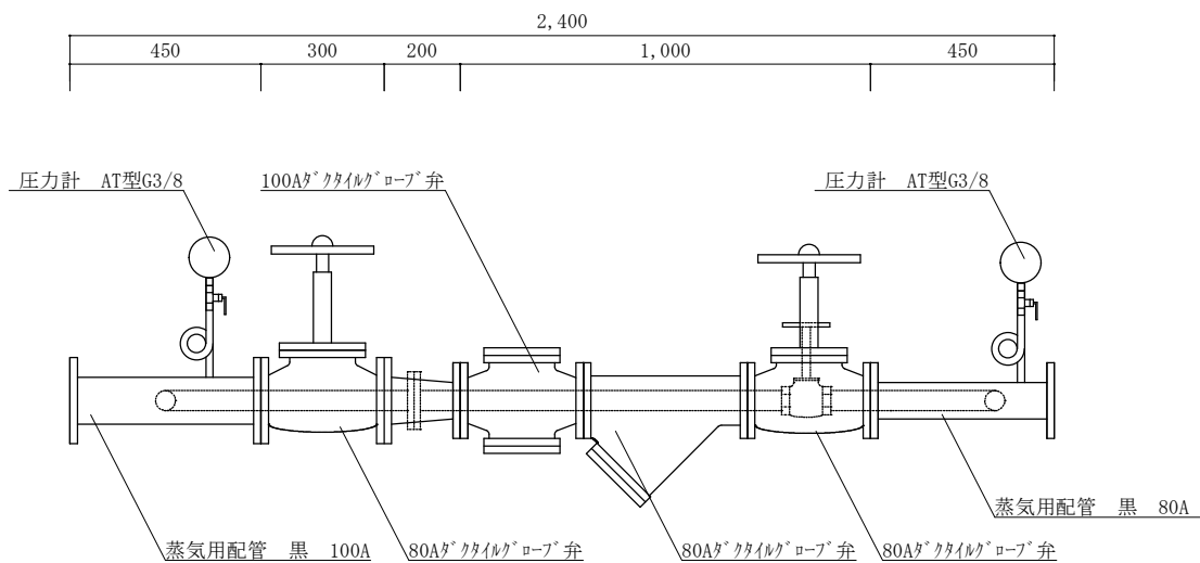
蒸気管詳細図（正面） S=1：20
