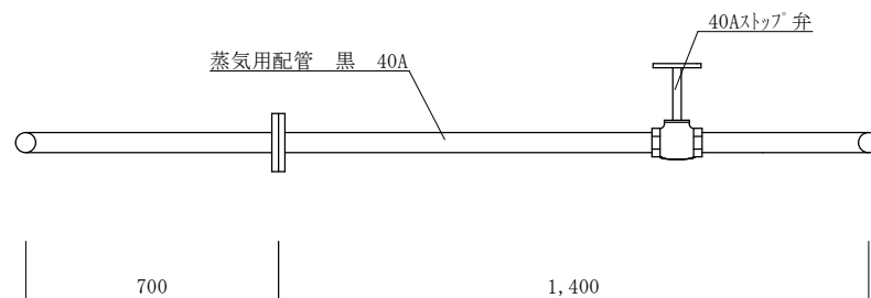
蒸気管詳細図（裏面） S=1：20
