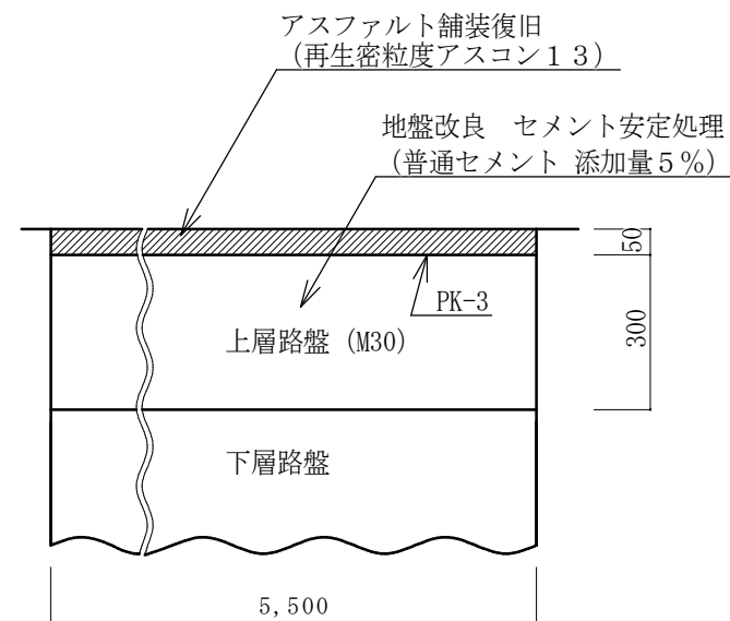
補修断面標準図 S=1/15
