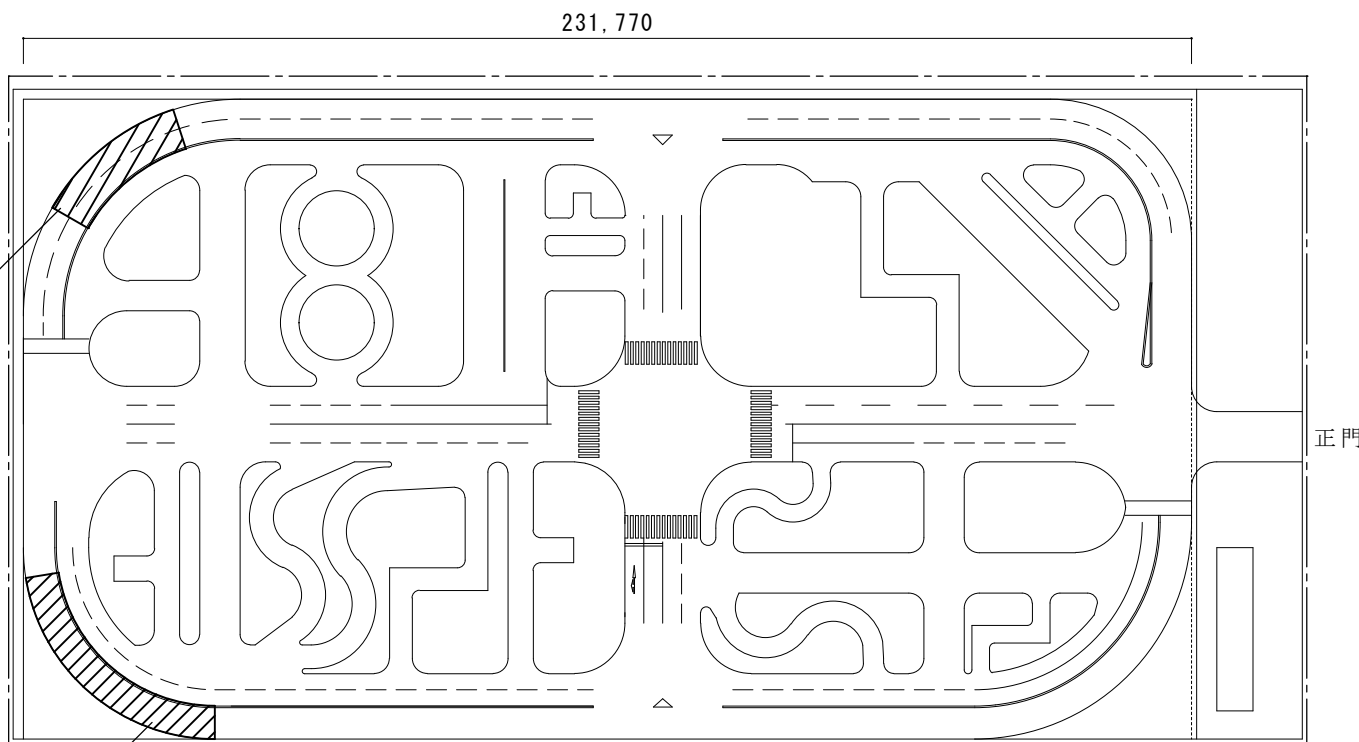
自動車訓練場配置図 S=1/1,500
