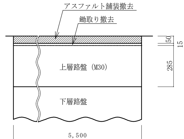
撤去断面標準図 S=1/15
