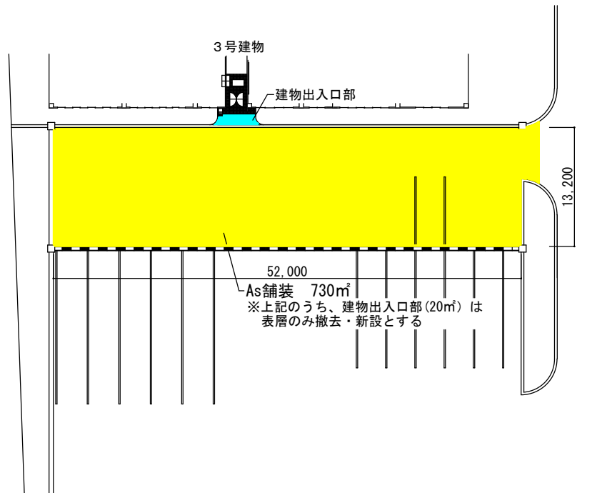
計画平面図（駐車場） S=1/600
