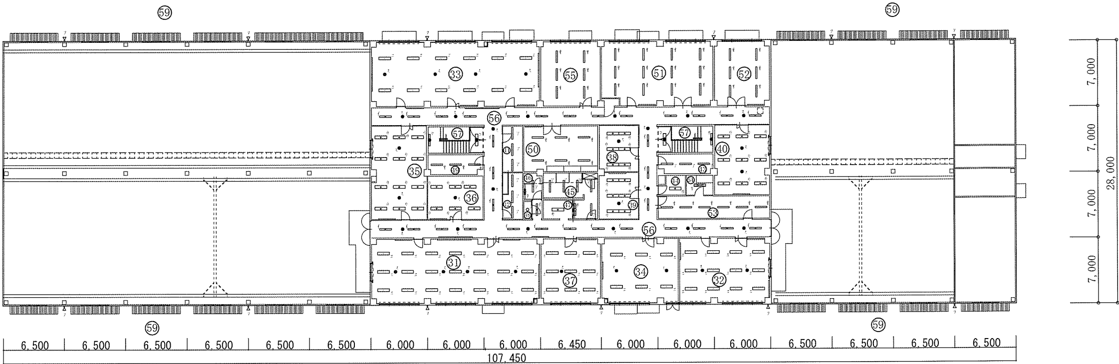
2 階照明器具配置図
