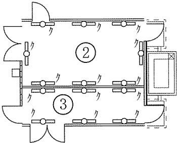
1 階東工区照明器具詳細配置図
