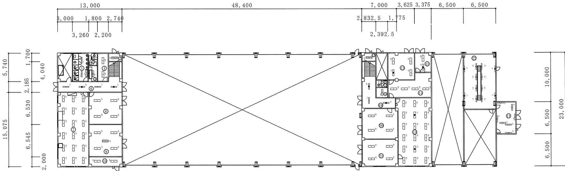
1階照明器具配置図
