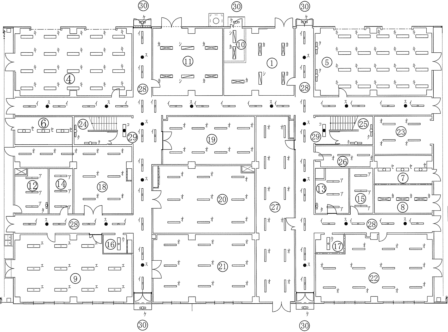
1 階東工区照明器具詳細配置図
