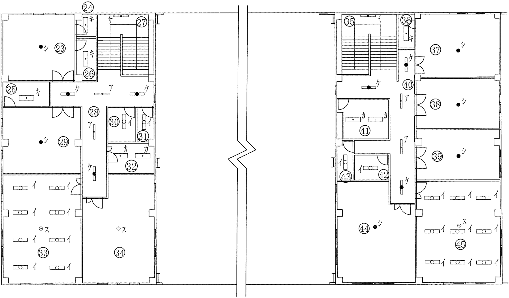
208号2階照明器具詳細配置図 1/200
