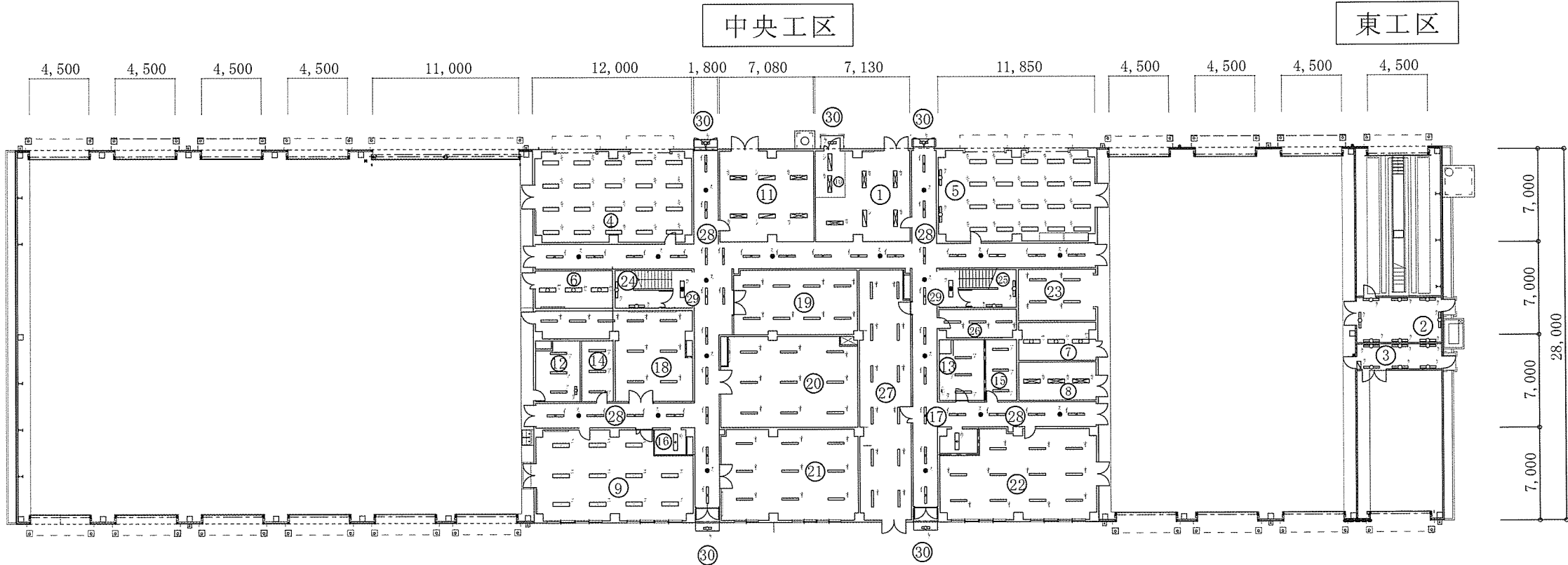
1 階照明器具配置図
