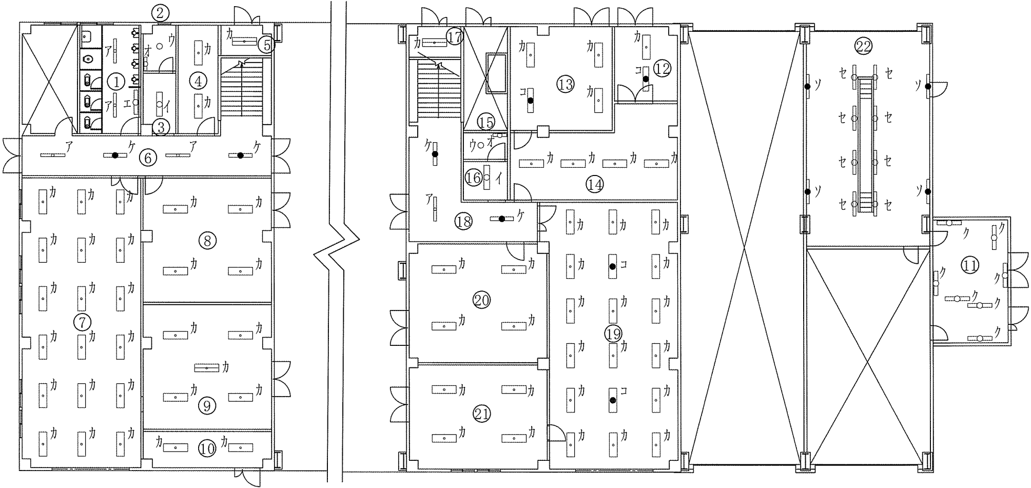
208号1階照明器具詳細配置図 1/200
