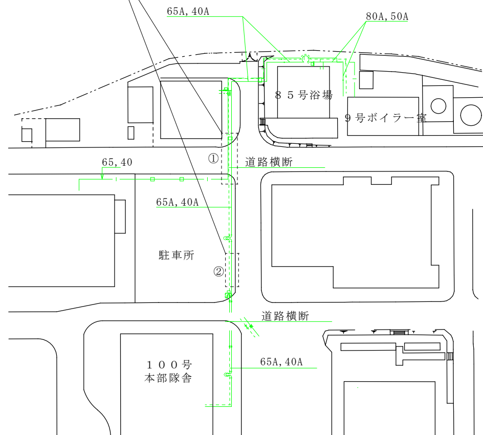
屋外配管図 S=1/600
