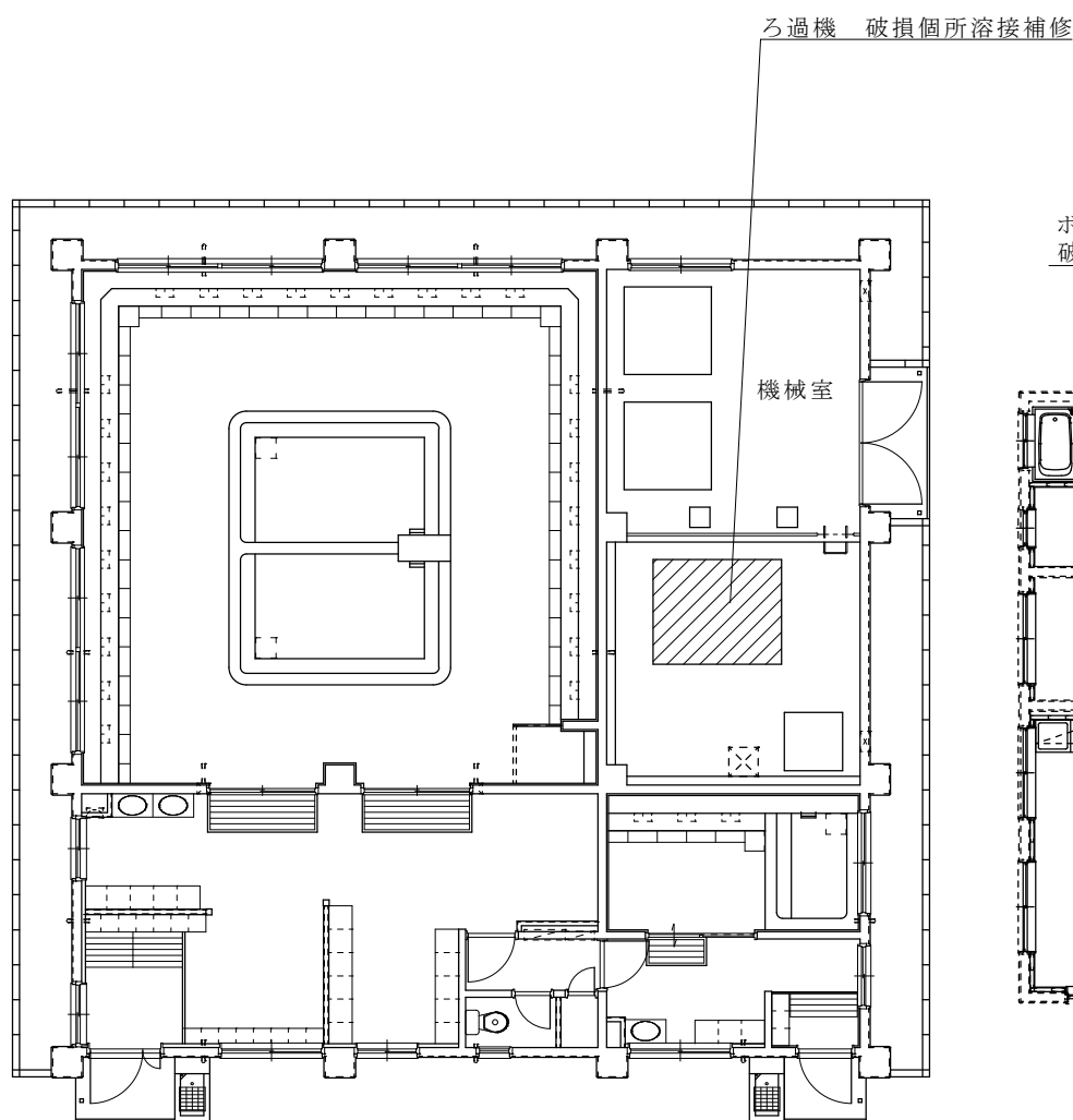
8 5号浴場 S=1/100
