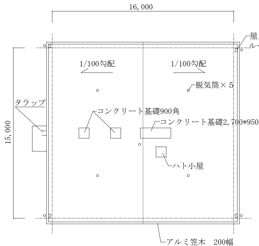
86号建物屋上平面図 S=1/200
