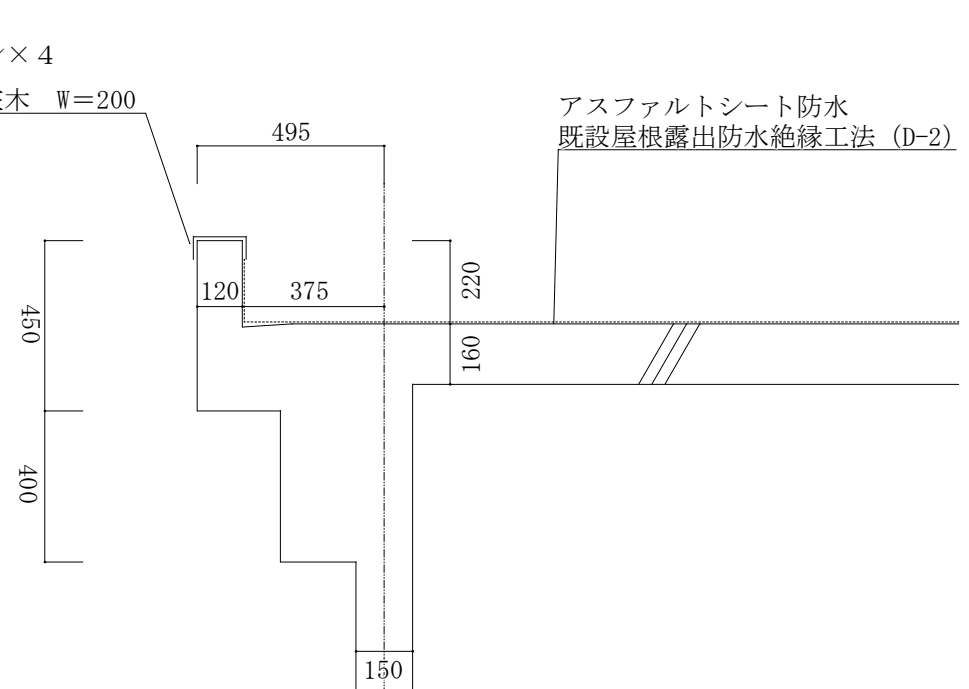
86号建物屋上断面図 S=1/20
