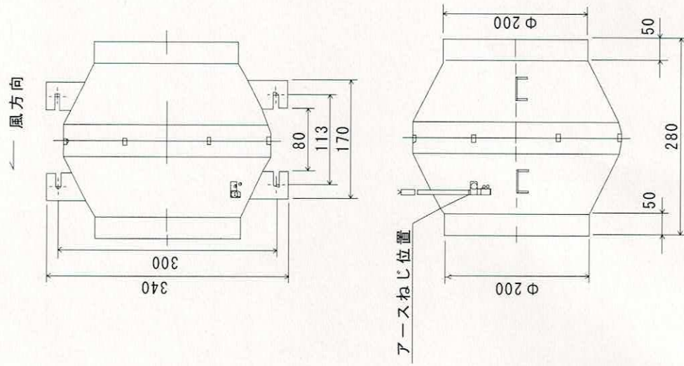
■外形図
