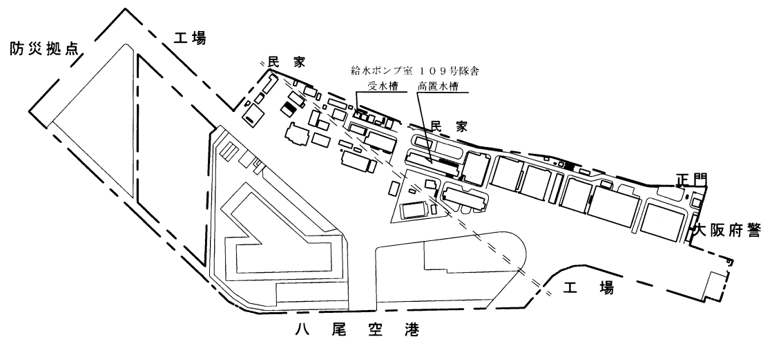
配置図
