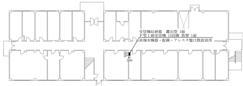
4号建物1階平面図 S=1/300
