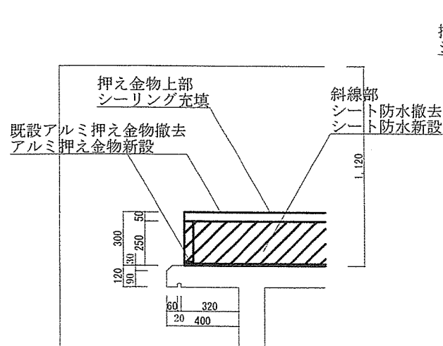
A～A' 断面図 1/30
