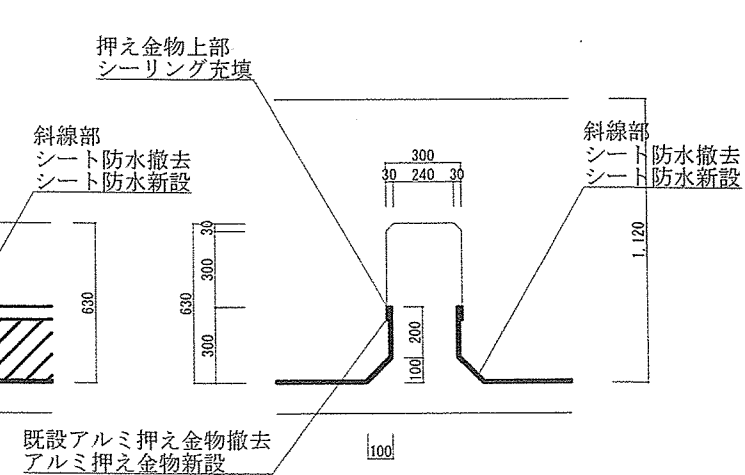
C～C' 断面図 1/30
