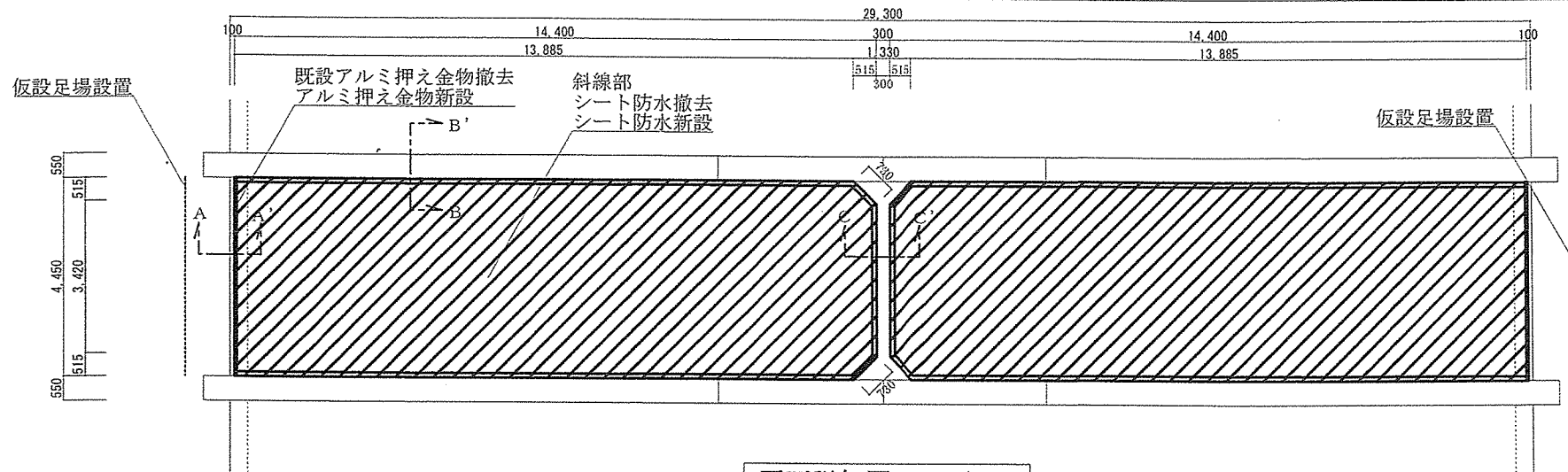
平面詳細図 S=1/150
