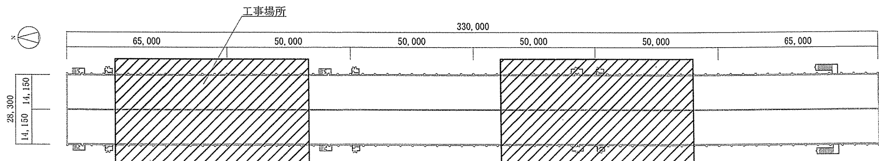
射撃場平面図 S=1/1,500
