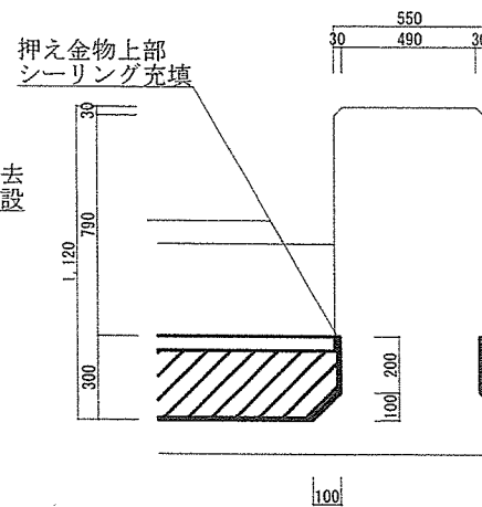
平面詳細図 S=1/150
