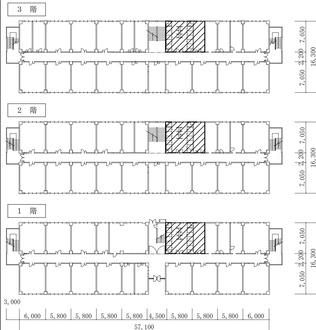
175号建物1～3階平面図
