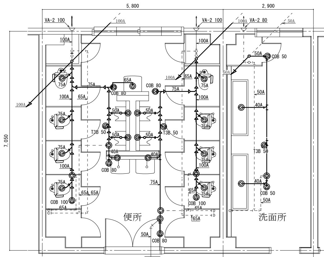
175号建物 3階便所・洗面所改修配管図 S=1/75
