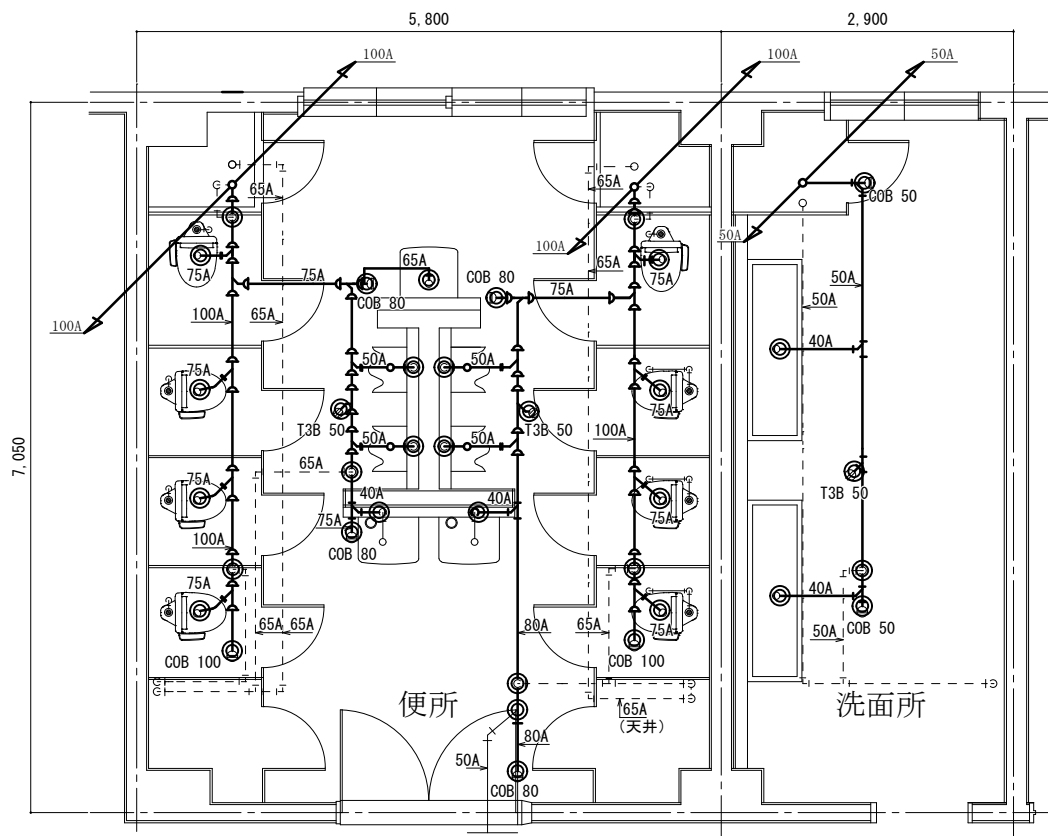
175号建物 2階便所・洗面所改修配管図 S=1/75
