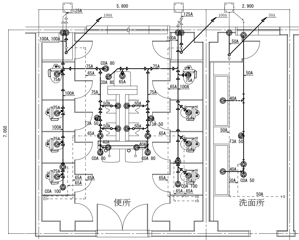
175号建物 1階便所・洗面所改修配管図 S=1/75
