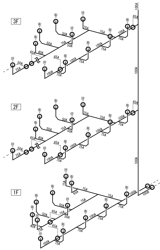
便所東側系統
