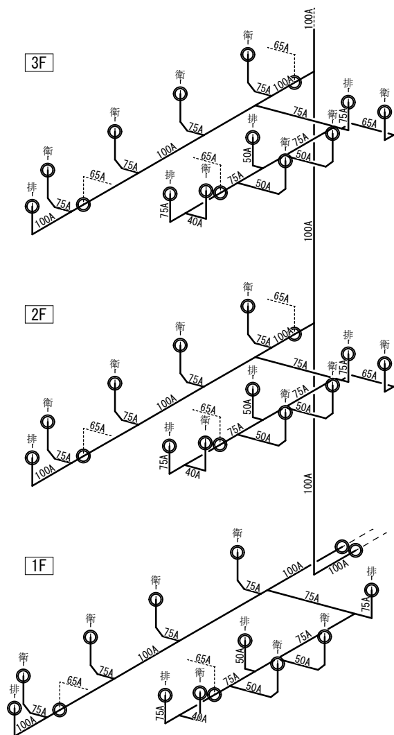
便所西側系統
