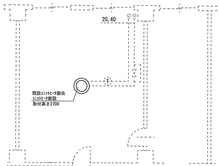
8号2階乾燥室平面図 S = 1 : 100
