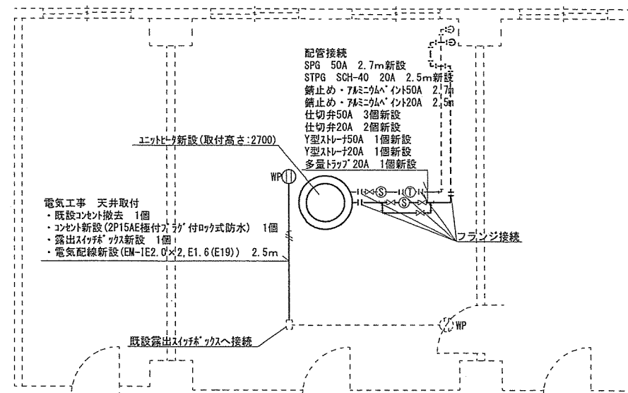
9号2・3階改修後乾燥室平面図 S=1:100
