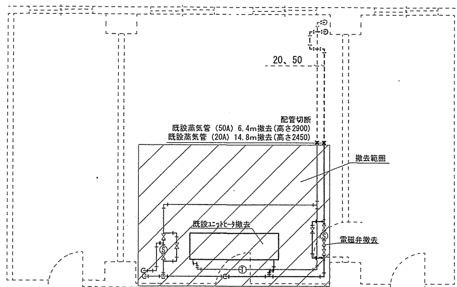
9号2・3階改修前乾燥室平面図 S=1:100
