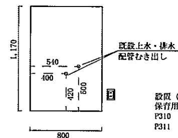
洗面台詳細図 (既設CB)
