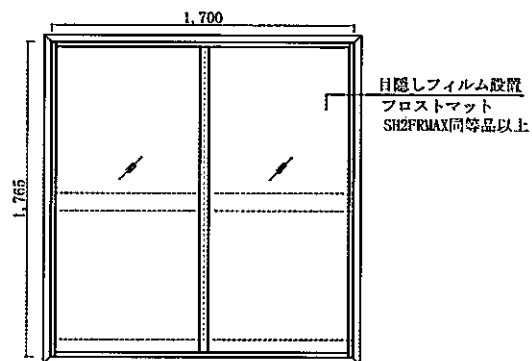
詳細図 (AW3)
