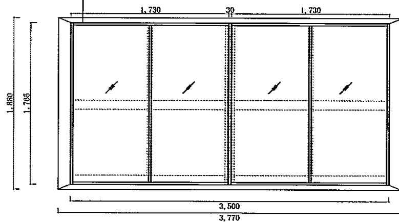
詳細図 (AW1)
