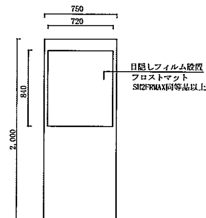
詳細図 (AW2)
