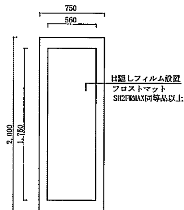
詳細図 (AW4)
