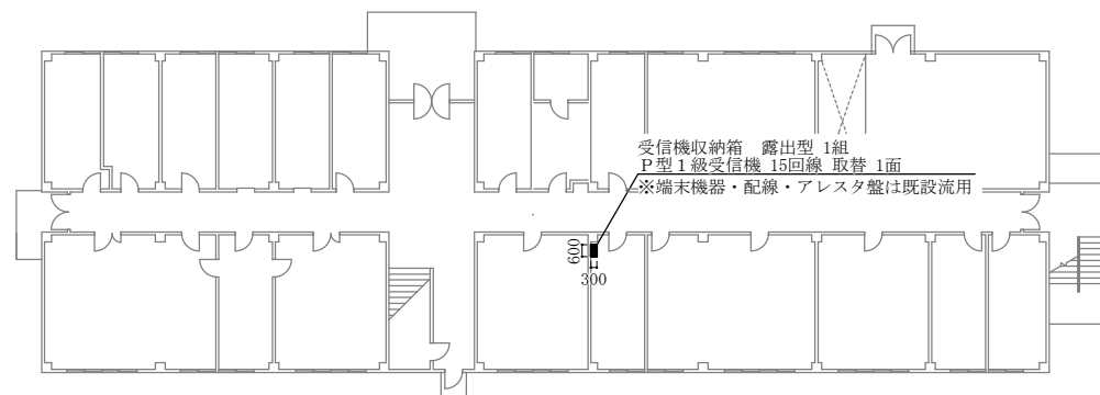
4号建物1階平面図 S=1/300
