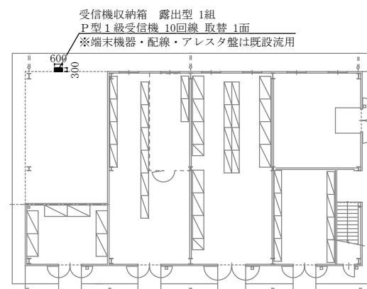
157号1階平面図 S=1/300
