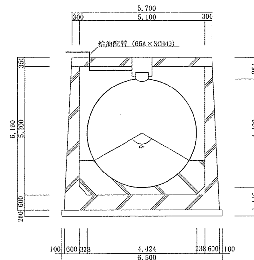
重油燃料タンク断面図
