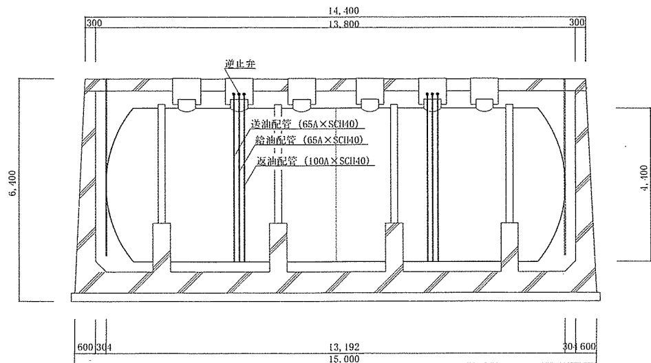
重油燃料タンク側面図
