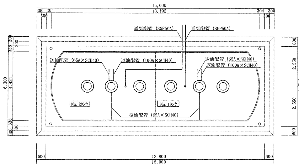
重油燃料タンク平面図
