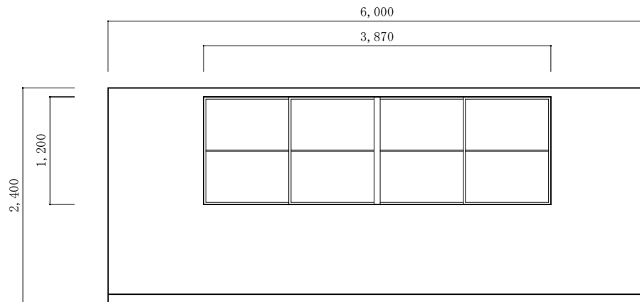
237号建物対象部屋A立面図 S=1：60
