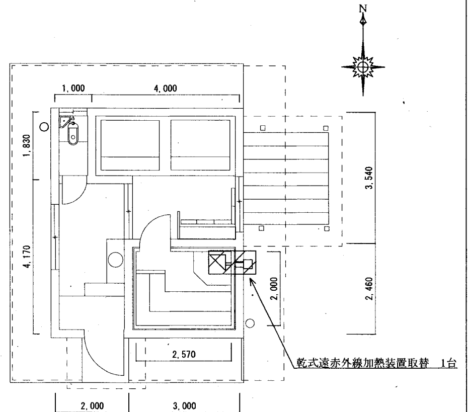
189号建物平面図 S=1/100
