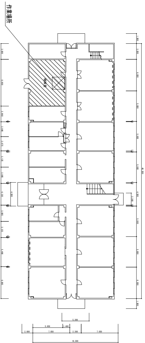
77号建物 1階平面図
