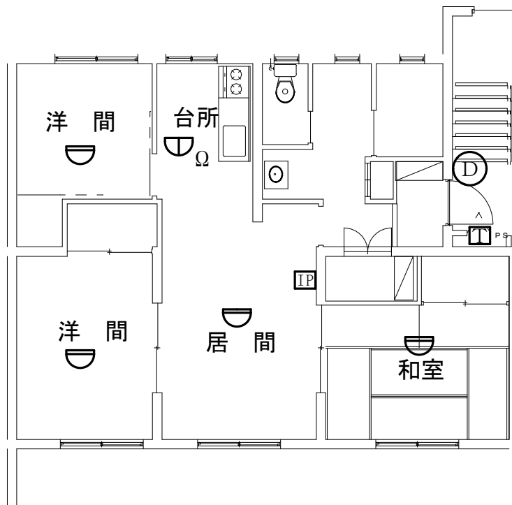
大桑宿舎D棟屋内消防設備配置図
