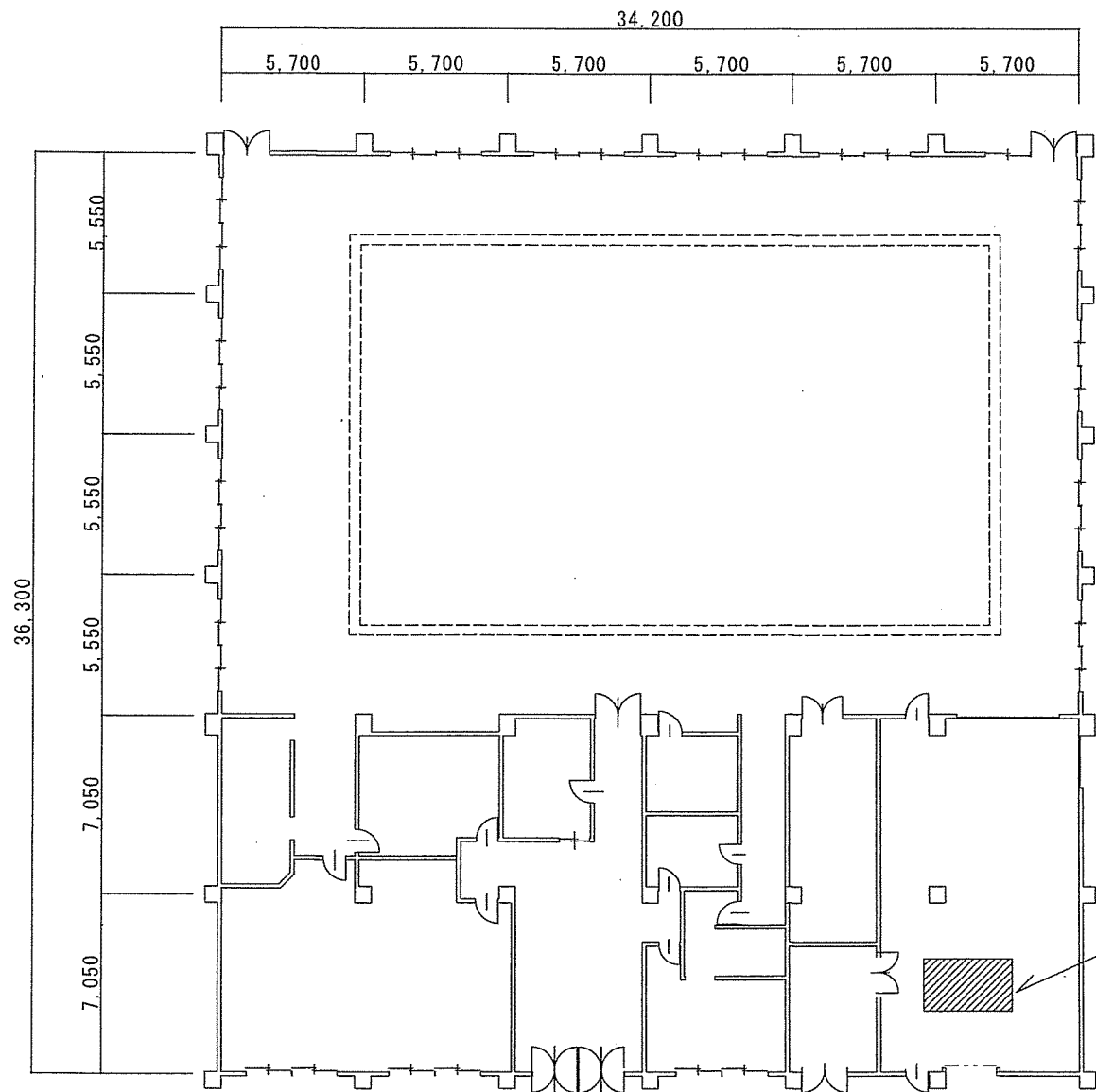
146号建物平面図 S-1/200
