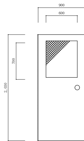
扉詳細立面図 (施工後) S=1:30
