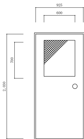
扉詳細立面図 (施工前) S=1:30
