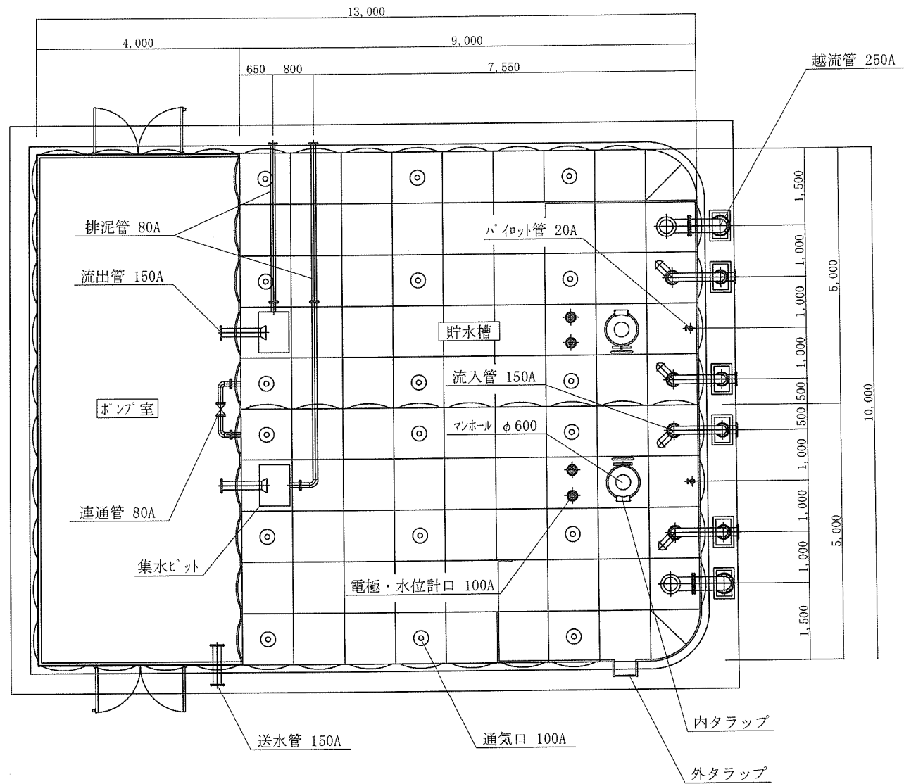
平面図 S=1/100
