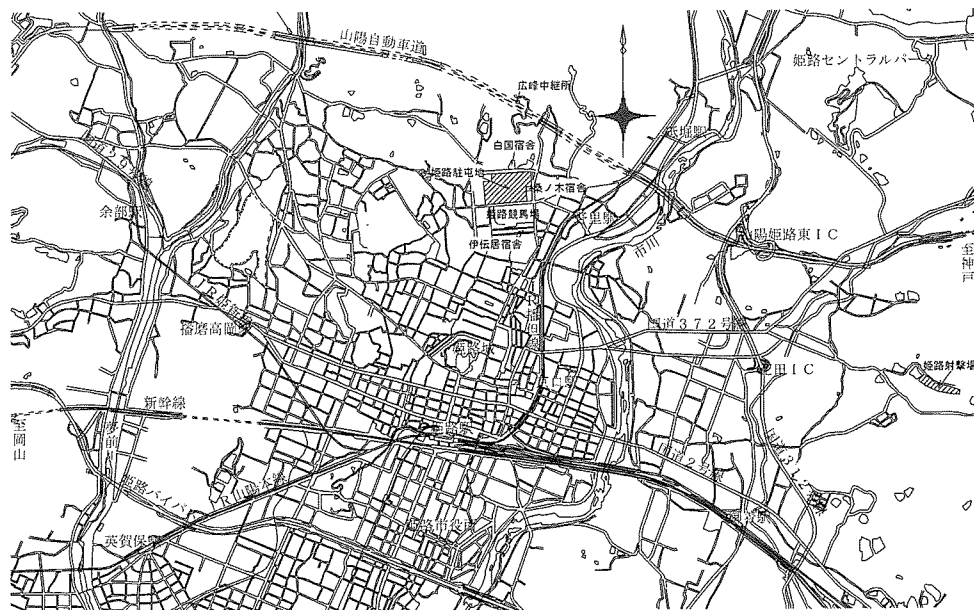
案内図 S=1:100,000
