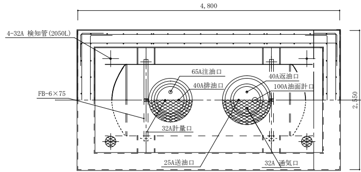
地下タンク平面図 S=1:100
