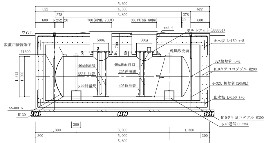
地下タンク断面図 S=1:100
