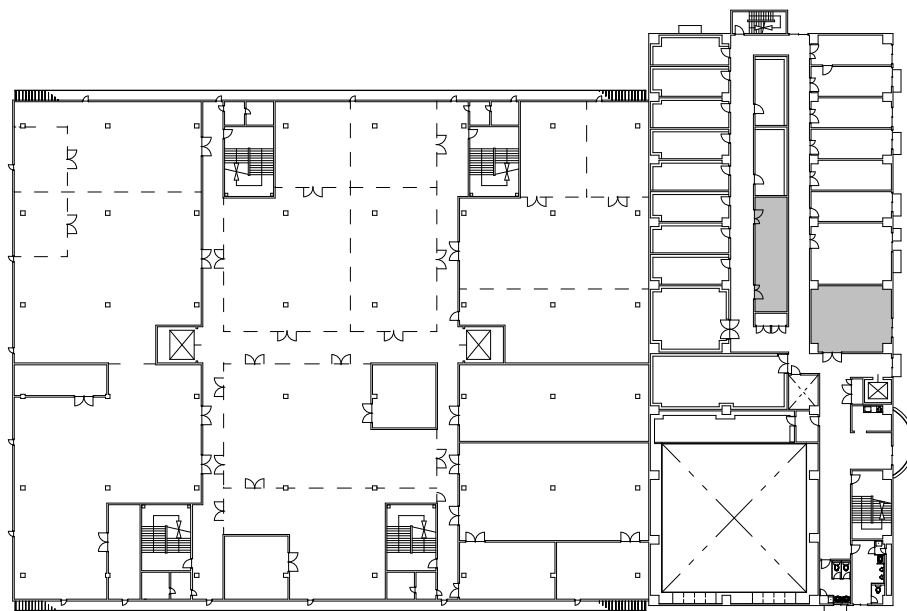
138号建物2階平面図 S=1/700
