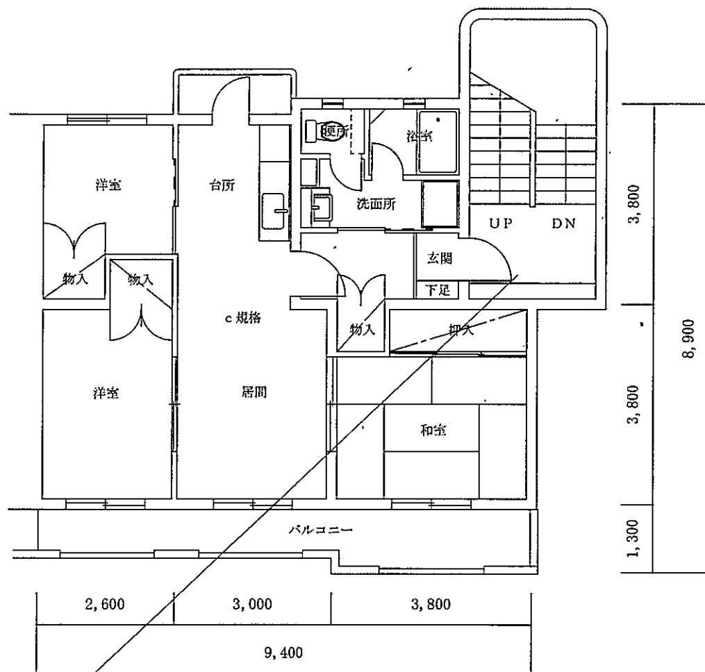
宿舎（善通寺町）平面図 S = 1/100
