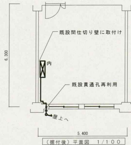
(据付後)平面図 1/100
