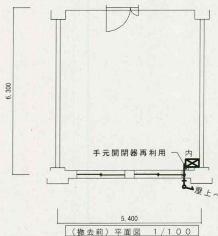
(撤去前)平面図 1/100
