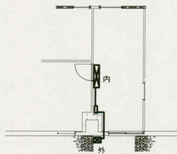
(撤去前)平面図 1/100
