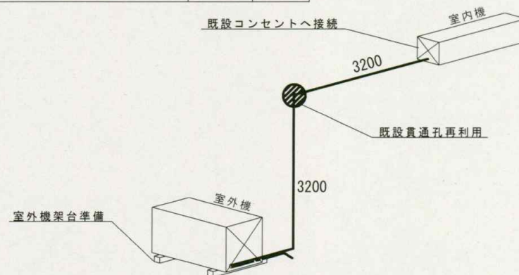
新設配管図（アイソメ図）
