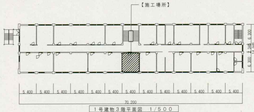
1号建物3階平面図 1/500
