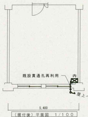
(据付後)平面図 1/100
