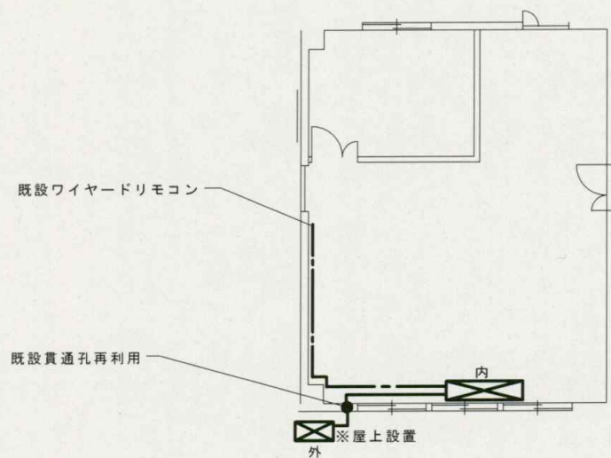
（据付後）平面図 1/100
