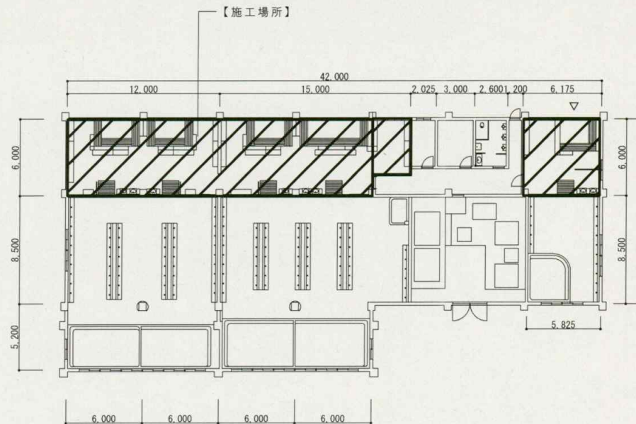
200号建物 平面図 1/500
