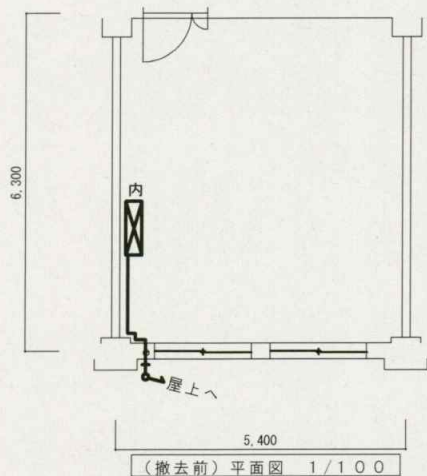
(撤去前)平面図 1/100
