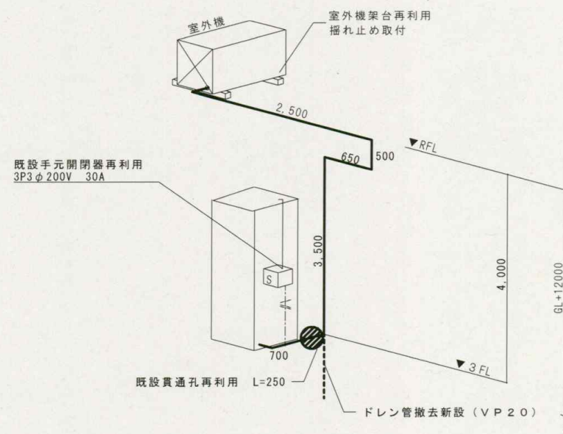
新設配管図 (アイソメ図)
