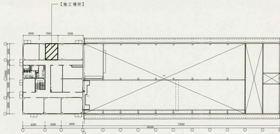
265号建物2階平面図 1/500
