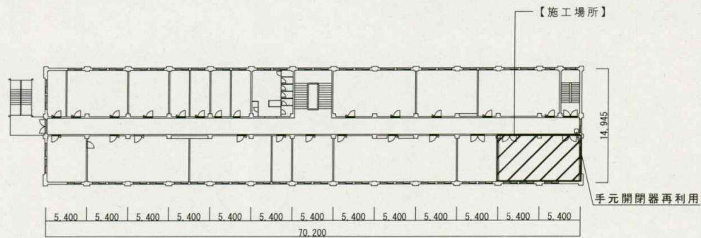
1号建物2階平面図 1/500
