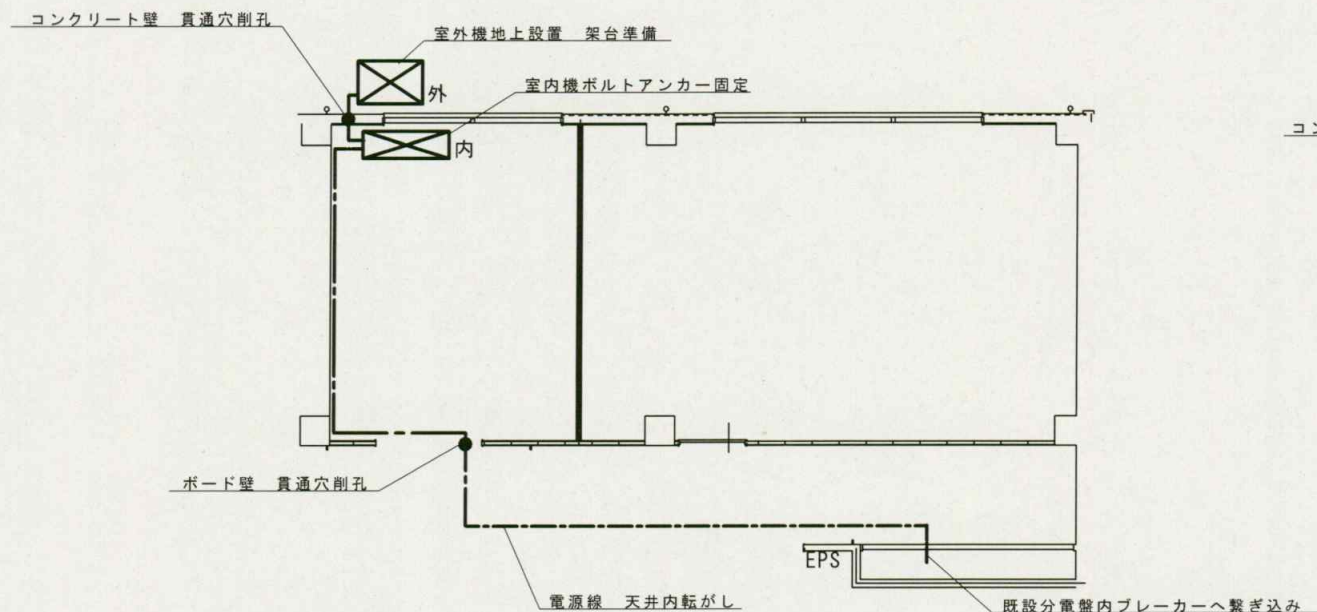
(据付後)詳細図 1/100
