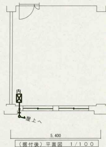
(据付後)平面図 1/100
