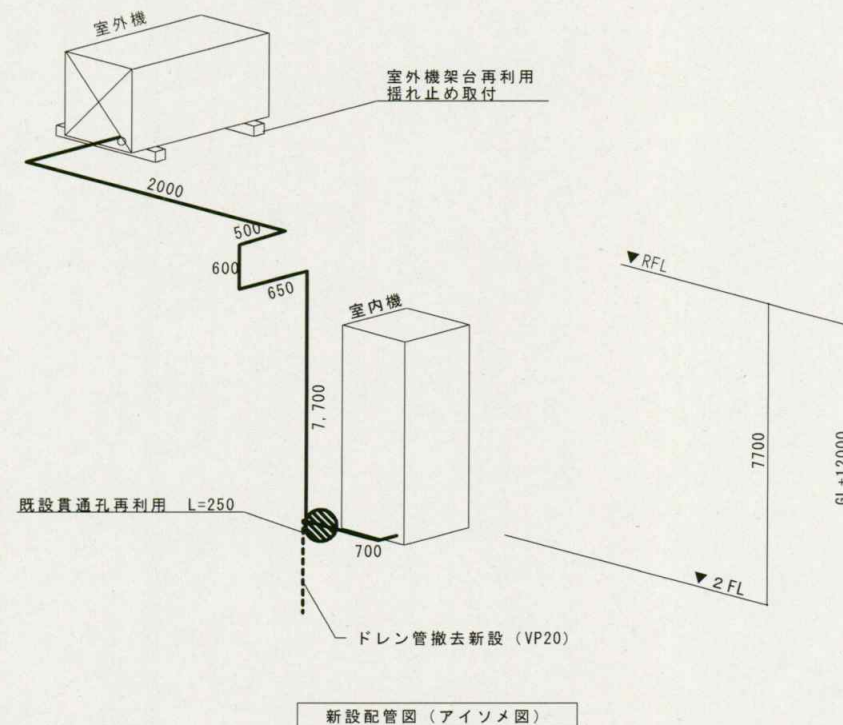
新設配管図（アイソメ図）
