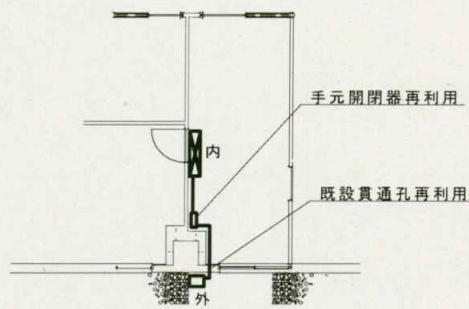
(据付後)平面図 1/100
