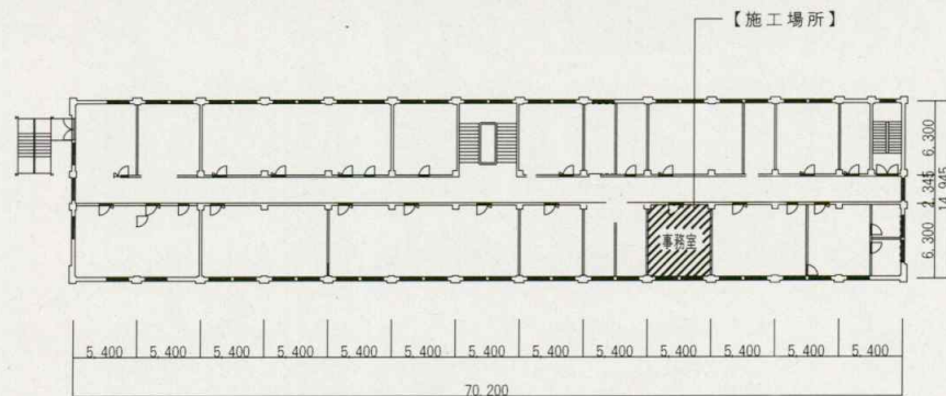
1号建物3階平面図 1/500
