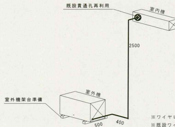
新設配管図（アイソメ図）
