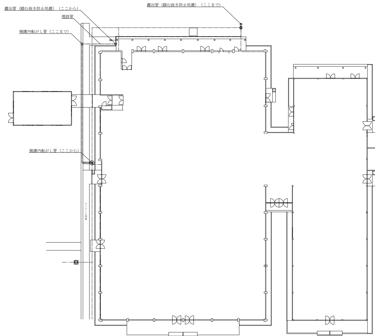
203号建物回り配管図 S=1:300
