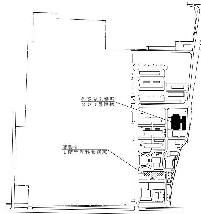
駐屯地配置図 S = 1 : 6,000
