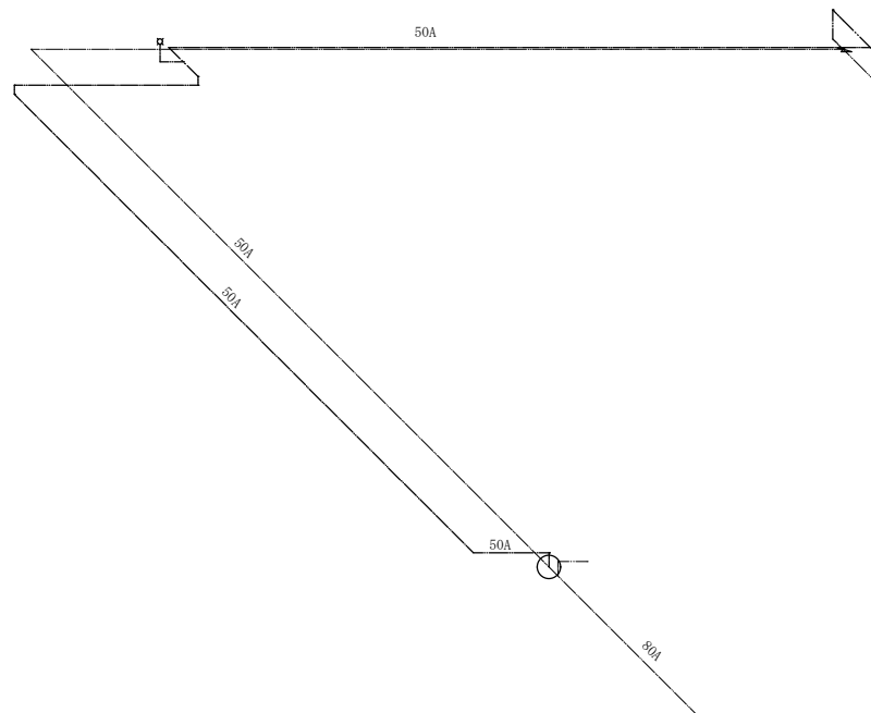
203号建物回り配管アイソメ図 S=1:200
