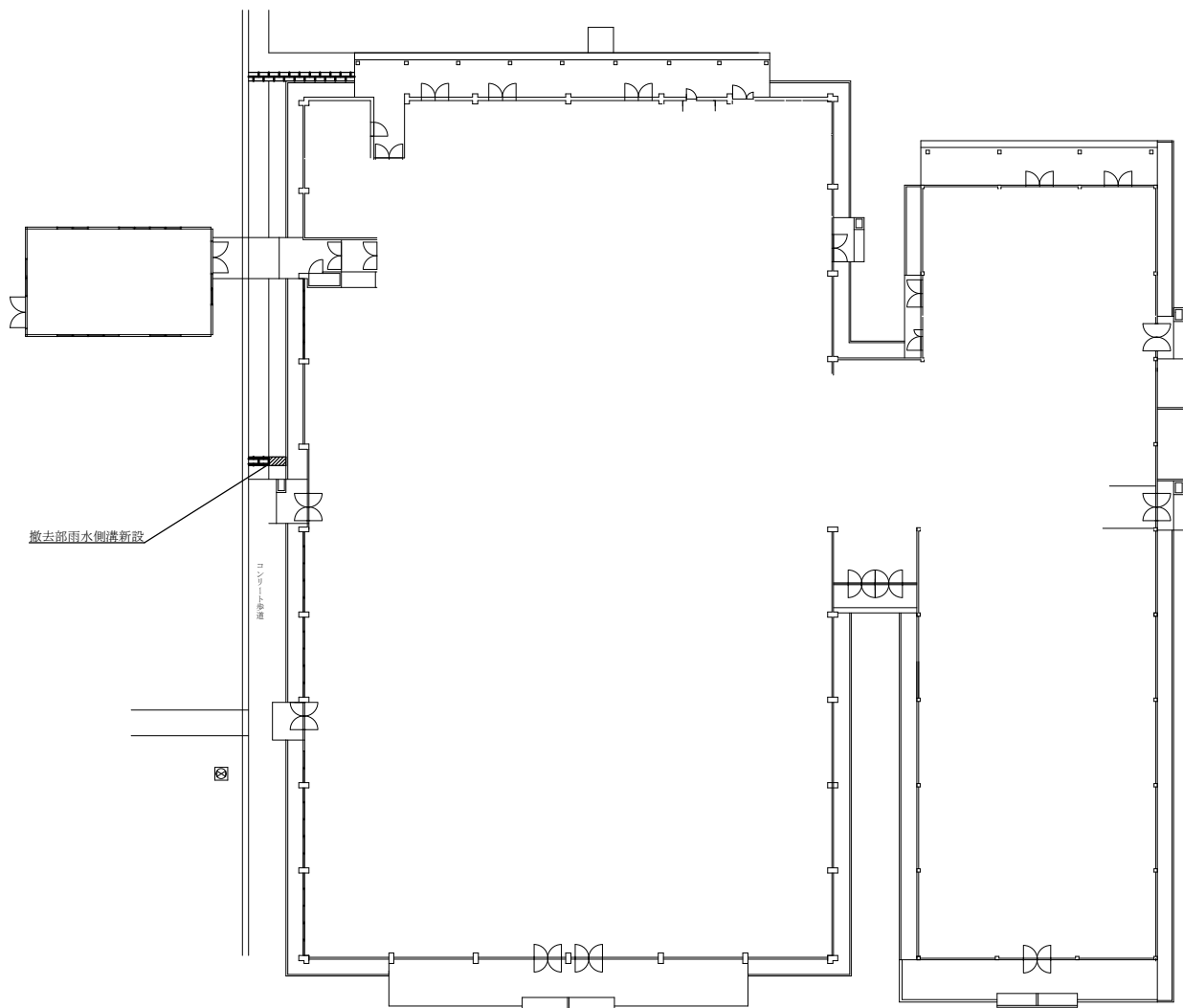
203号建物回り平面図 S=1:300
