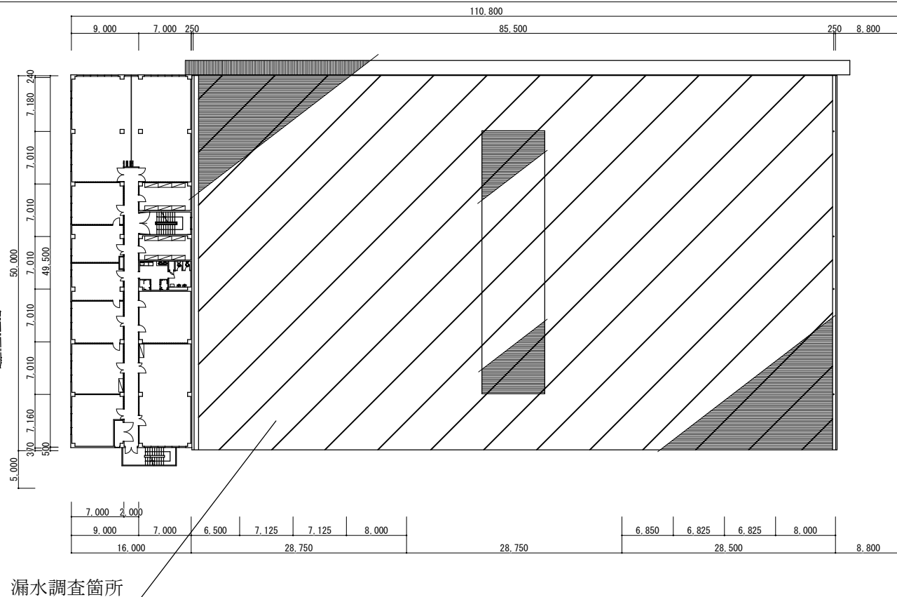
E格納庫 (58号建物) 屋根伏図 S=1/500
