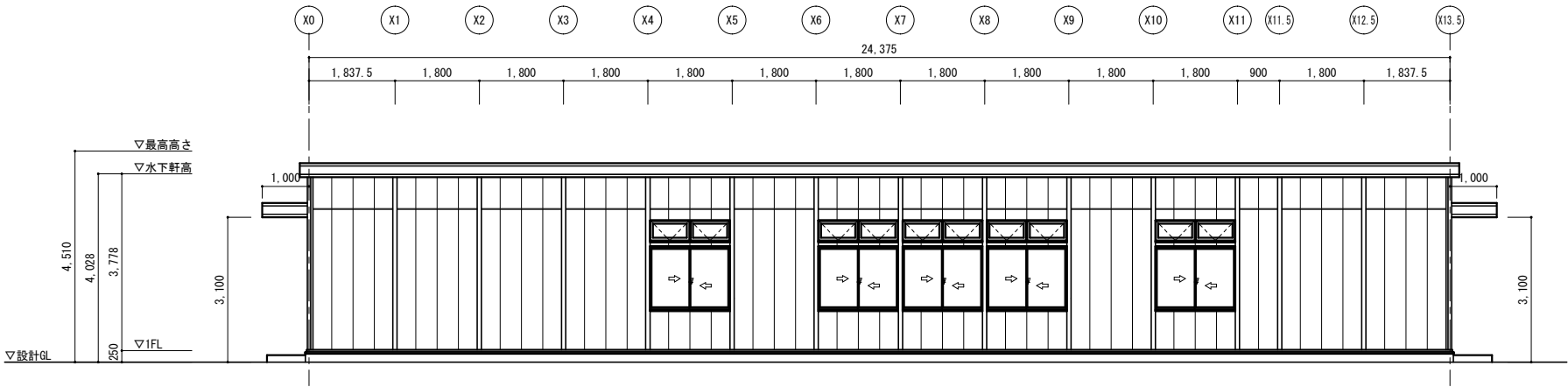
Y O 通立面図 S=1:100
