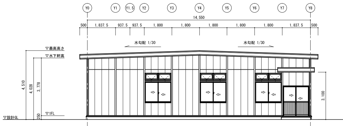
X 1 3. 5 通立面図 S=1/100
