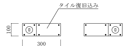
フロアヒンジ平面図 S=1/15
