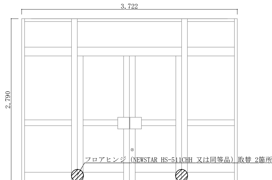
4号建物建具正面図 S=1/40
