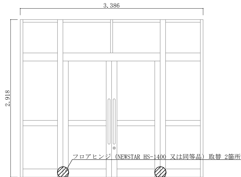
3号建物建具正面図 S=1/40
